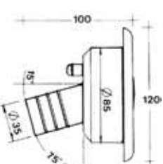
D Foro uscita Ø 35 mm
