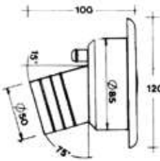
F Foro uscita Ø 50 mm
