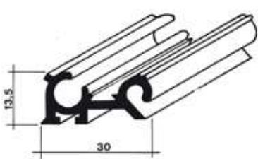
41218.AA Profilo Portafinestra + oscurante
