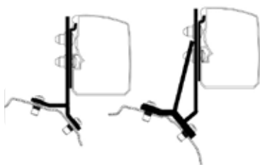
Kit staffe Thule 3200 per Ford Transit - Tourneo Custom Minivan passo corto e lungo
