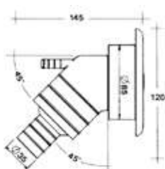
A Foro uscita Ø 35 mm
