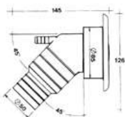
C Foro uscita Ø 50 mm
