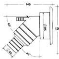
B Foro uscita Ø 40 mm
