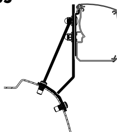
Kit staffe Thule 3200 VW Transporter 2025 e Ford Custom V710
