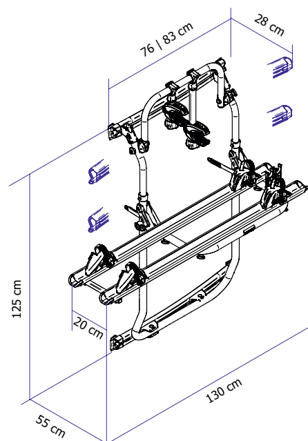
Thule Elite Van XT - Black Sprinter > 2006 + VW Crafter < 2016 (art. su ordinazione)
