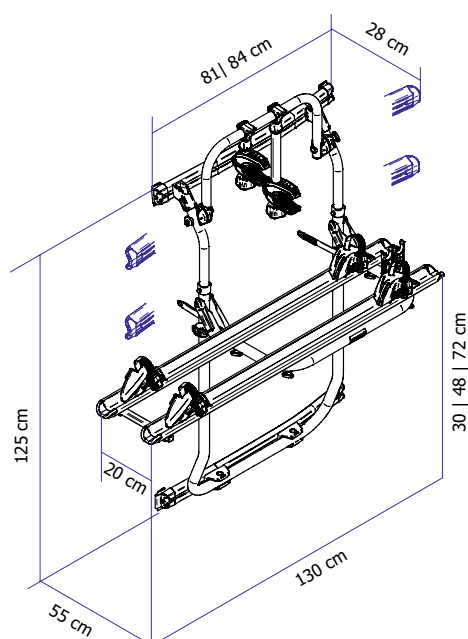
Thule Elite Van XT - Black Ford Transit H3 (art. 81092.FD)
