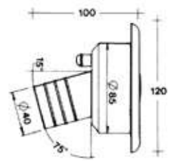
E Foro uscita Ø 40 mm
